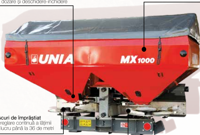
Mecanism de împrăștiere realizat din oțel inoxidabil
